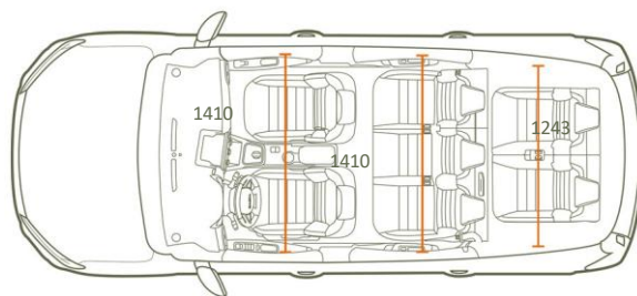
POGLED ODOZGO - SA 7 SJEDIŠTA
