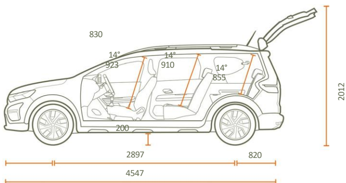
POGLED BOČNO - SA 7 SJEDIŠTA
