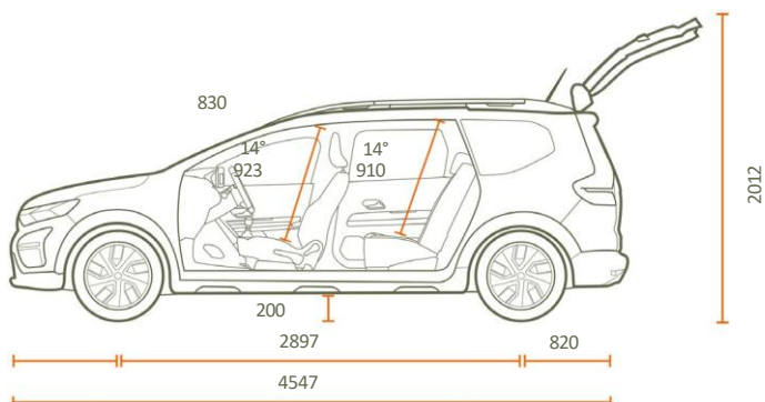
POGLED BOČNO - SA 5 SJEDIŠTA
